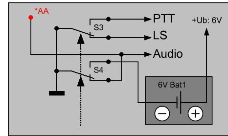
Variante mit Batterie und Lautsprecherabschaltung
