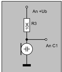
Alternativ mit Elektretkapsel
